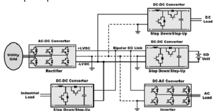
Fig. 1. Bipolar dc link.
